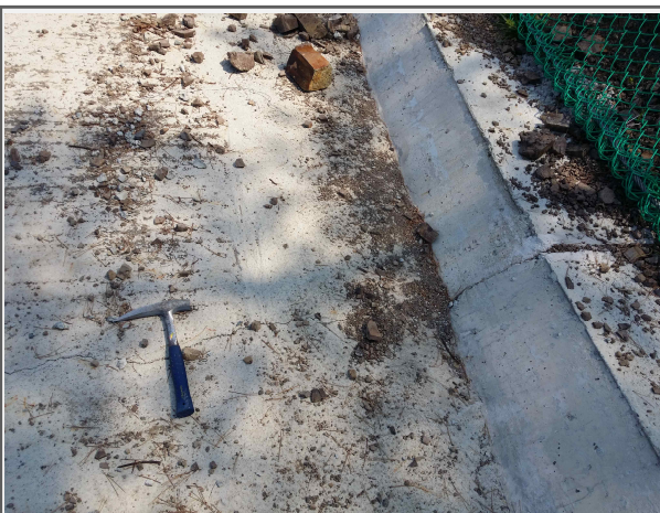
⑤ Sta.6+400부근(상주) 20m 소단 중방향 균열 발생
