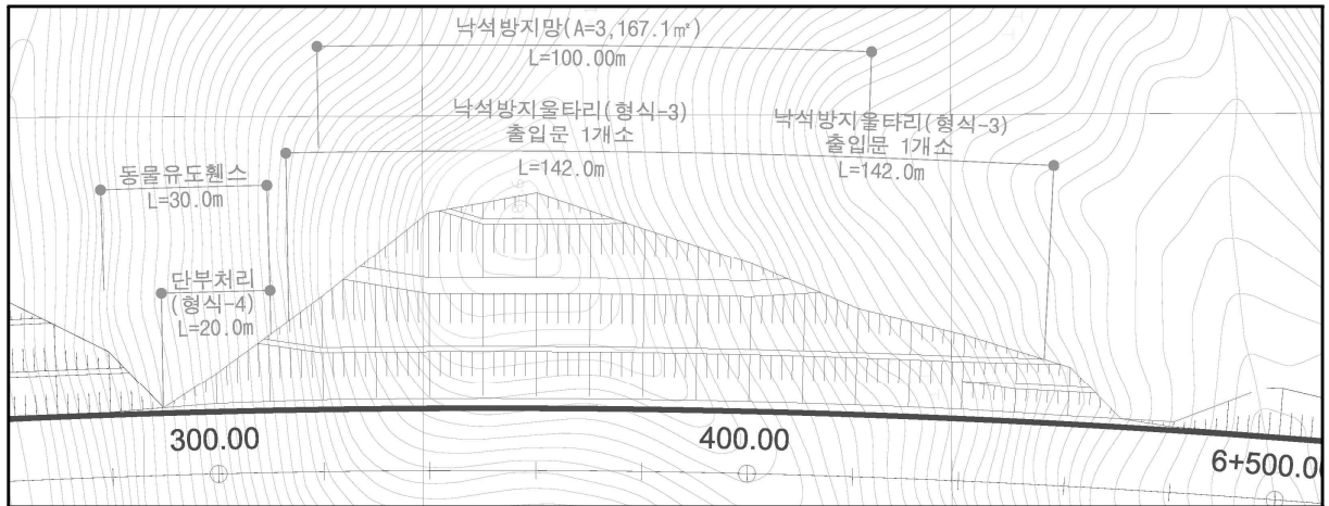
【Sta.6+280~6+480 평면】
