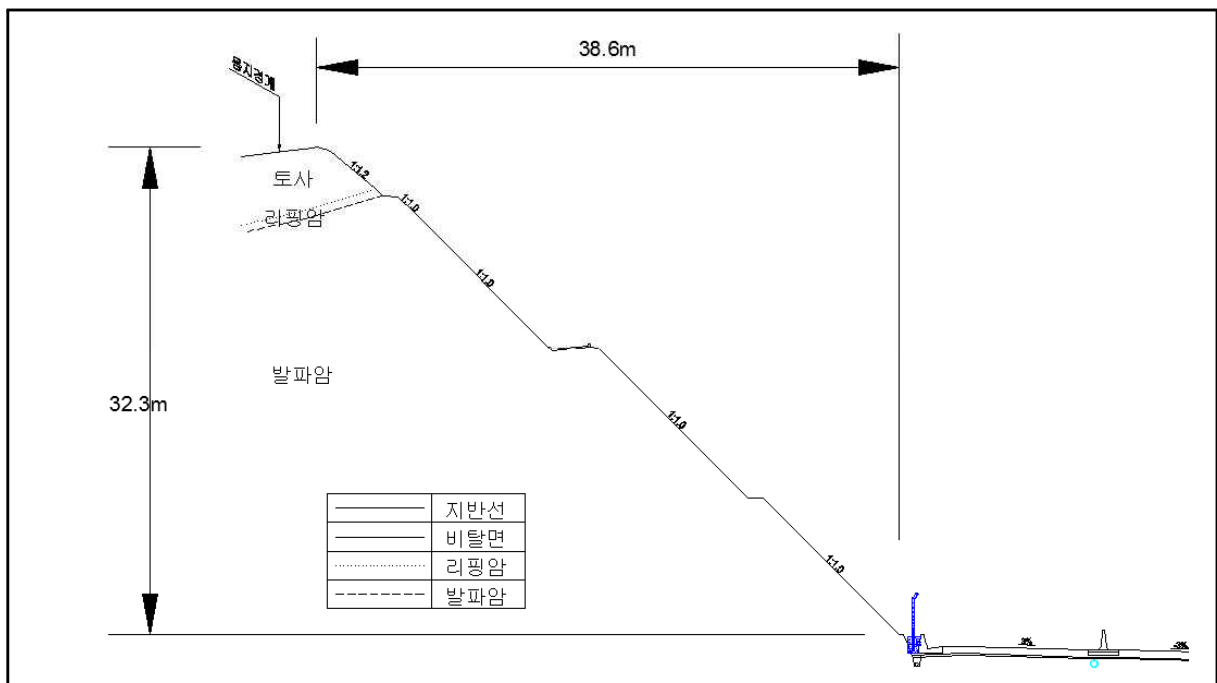
【대표단면 Sta.6+360(상주)】
