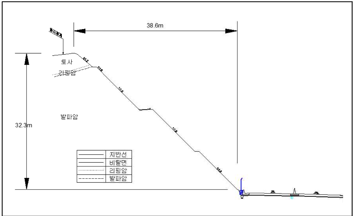
【대표단면 Sta.6+360(상주)】
