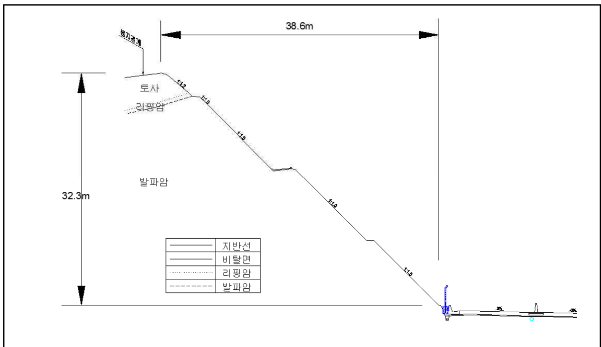
【대표단면 Sta.6+360(상주)】
